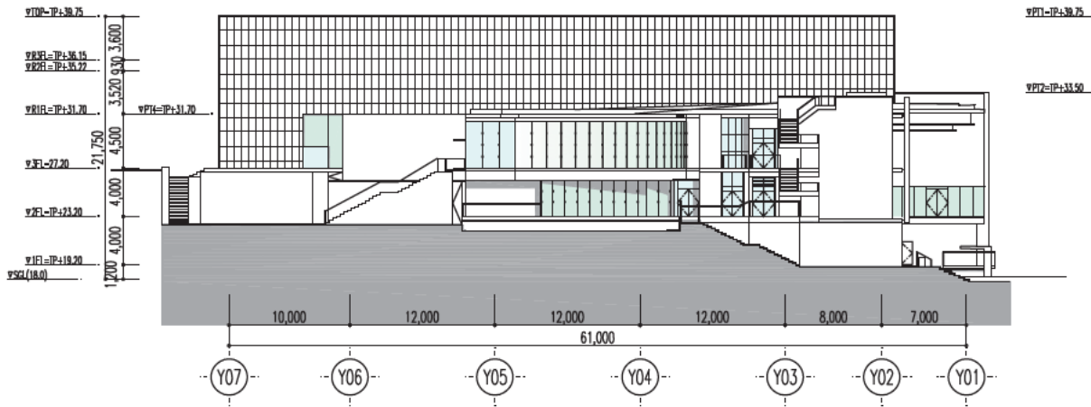
4. 北東面立面図
