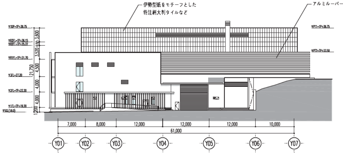
3. 南西面立面図
