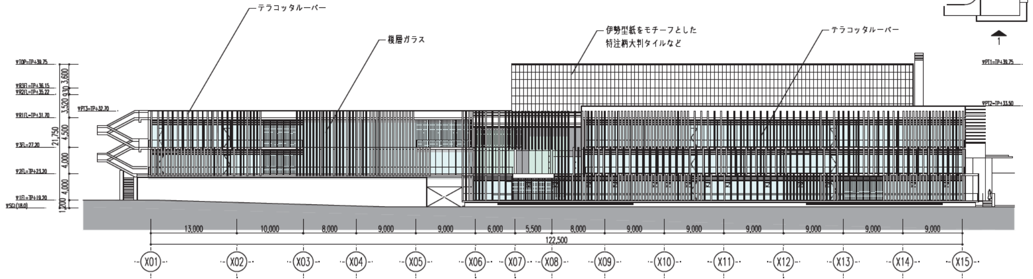
1. 北西面立面図
