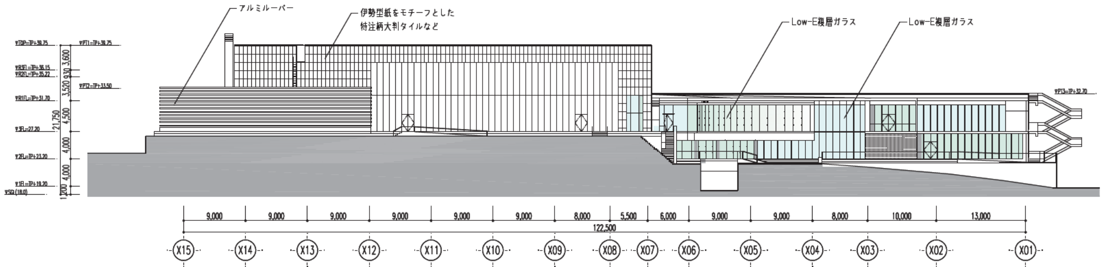
2. 南東面立面図
