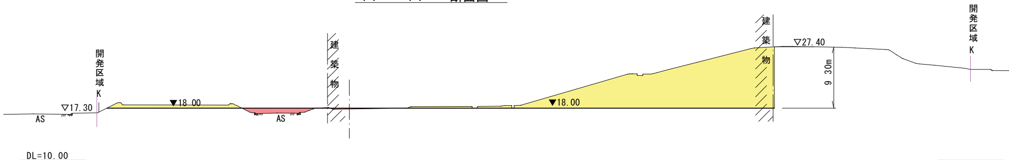
Y1 - Y1' 断面図 S=1:200
